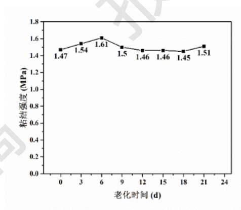
图 3 验证试验数据（样品 1，模拟室内环境）
