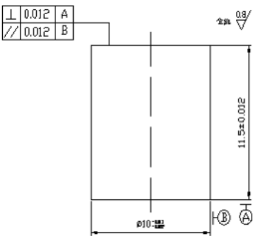
图 12 滑柱
